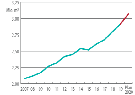
Entwicklung KVH-Produktion 2007–2020 laut Holzkurier-Erhebung
