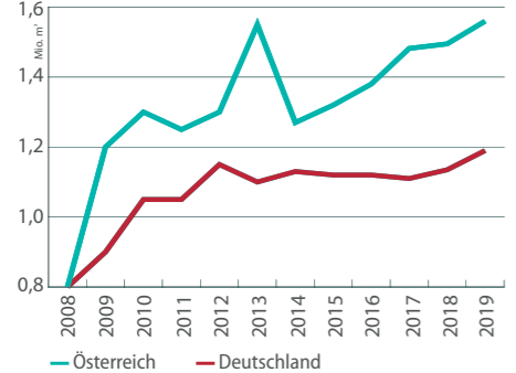
Entwicklung BSH-Produktion | 2008 bis 2019
