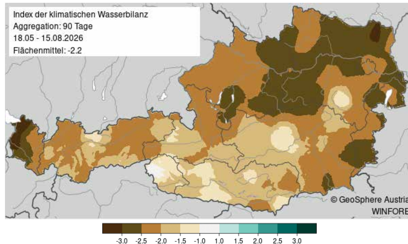
Abb. 1: Index der klimatischen Wasserbilanz Österreichs für den Zeitraum vom 18. Mai bis 15. August 2026 (Geosphere Austria: https://www.zamg.ac.at/incaanalyse/ ). Die Klimatische Wasserbilanz berücksichtigt sowohl Niederschlag als auch den atmosphärischen Verdunstungsanspruch. Bei Werten unterhalb von -2 wird von einer extremen meteorologischen Dürre ausgegangen.
